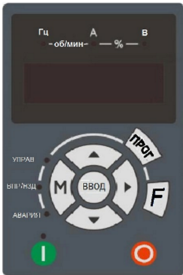
Внешний вид панелей управления преобразователей частоты АХ300
